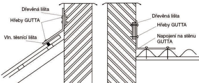
Schéma napojení na stěnu - boční
