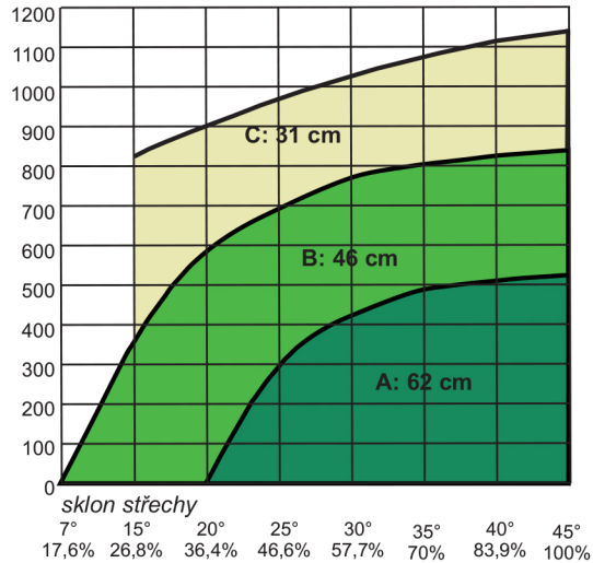
Závazná tabulka rozestupu lať
